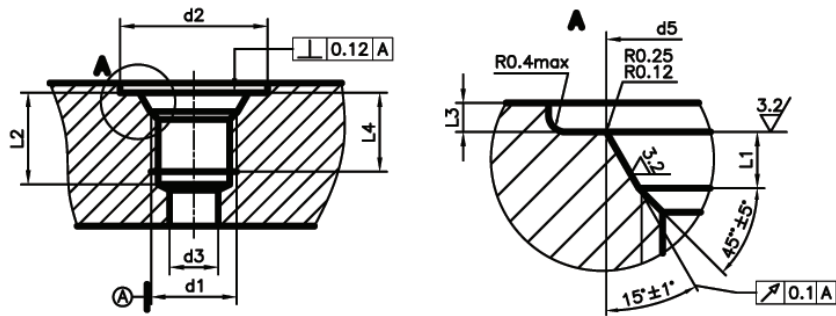
BS 5380 油口Port
