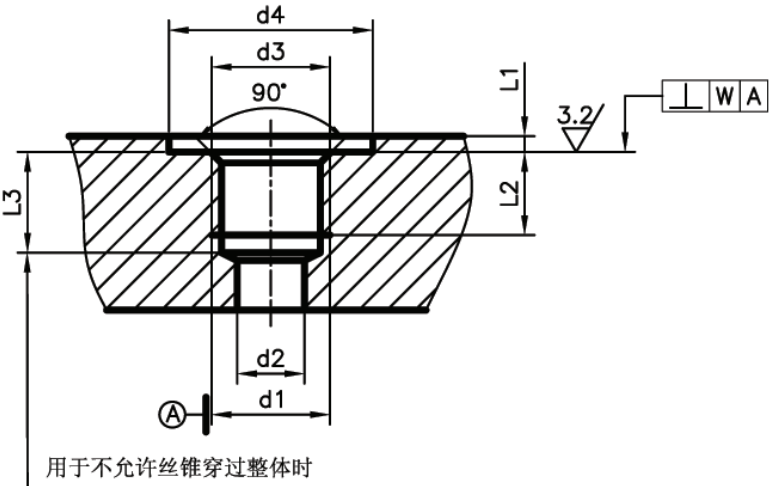
ISO 9974-1 油口Port
