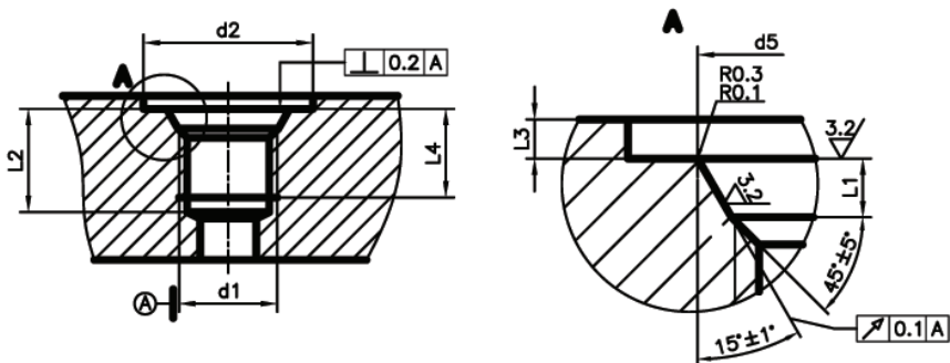
JIS B 2351 油口Port
