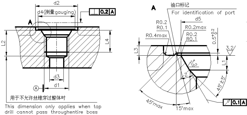
ISO 6149-1 油口Port
