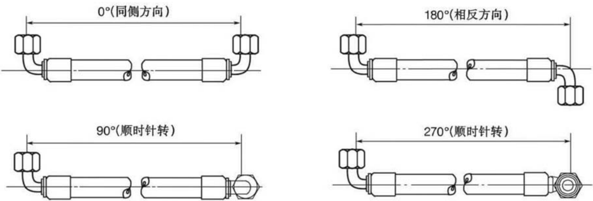
装配角允许误差 ±3°
