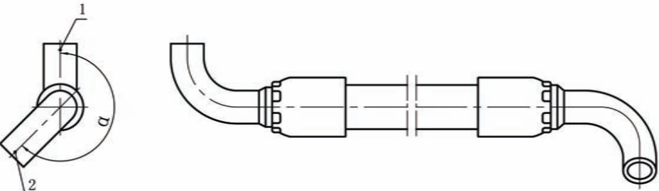
软管总成自然弯曲方向的规定
