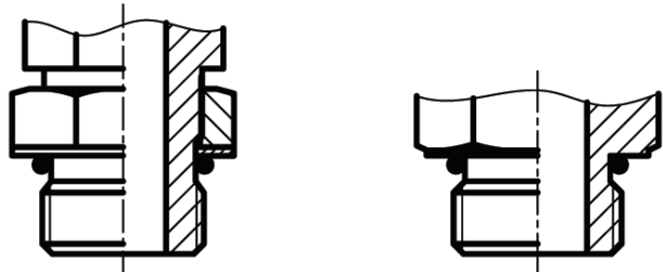
ISO 6149-2、ISO 6149-3 柱端stud end
