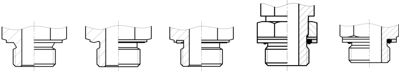
DIN 3852 A型柱端 DIN 3852 Type A
