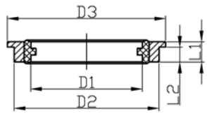
KDS 弹性密封垫
